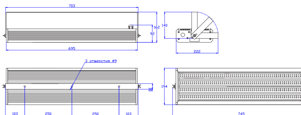
Светильник PROM 150 с креплением скоба
